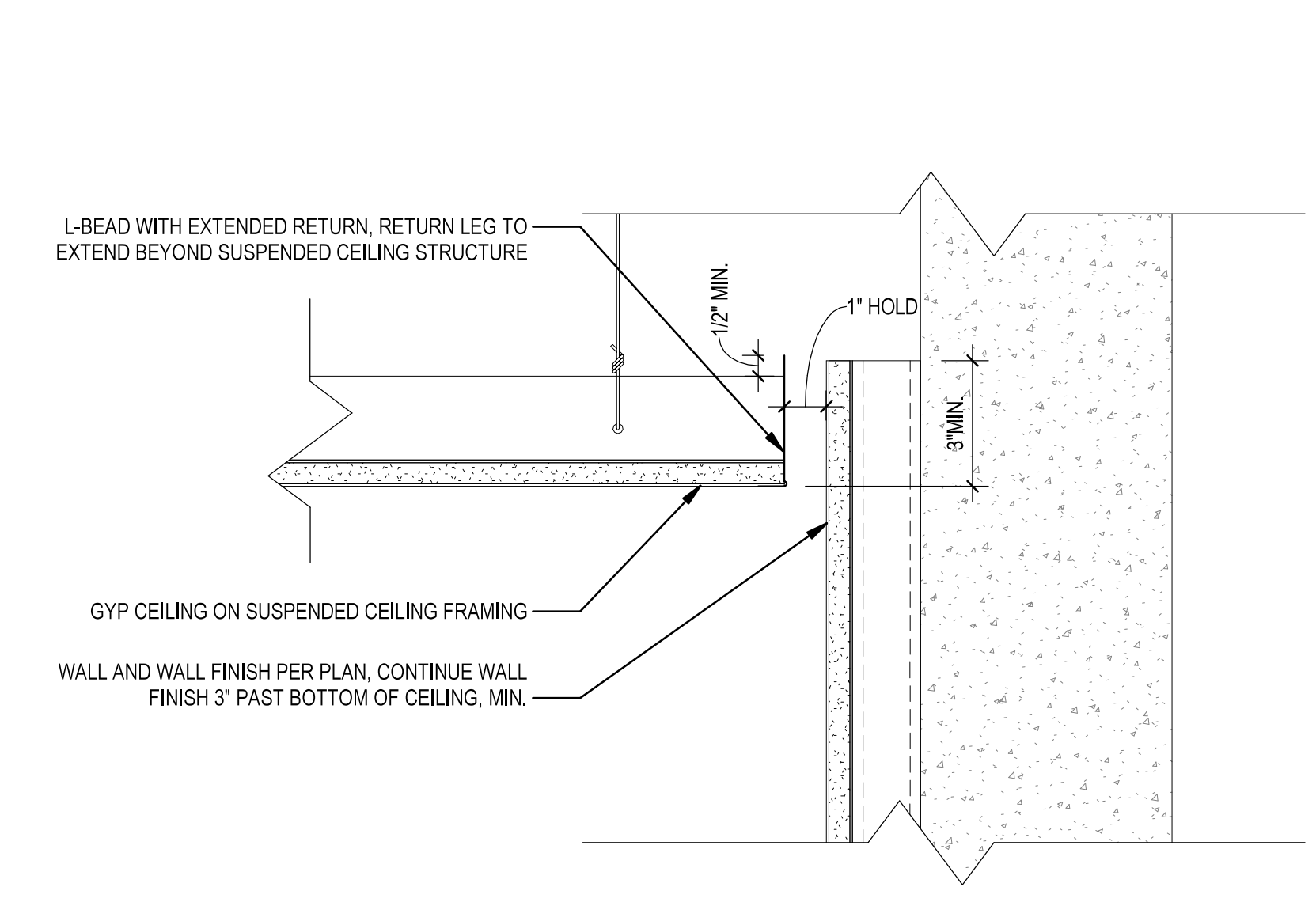
5 SECTION - ARCHITECTURAL PLENUM RETURN SLOT SCALE: 3" = 1'-0"
